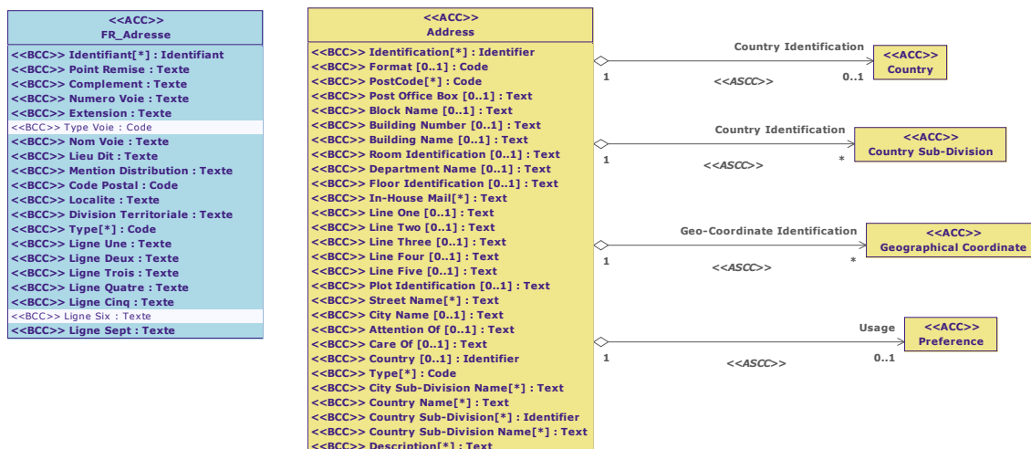
Diagramme de classe : Vue Adresse
