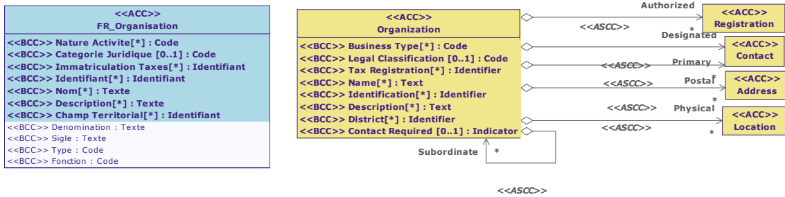
Diagramme de classe : Vue Organisation
