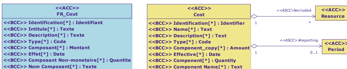
Diagramme de classe : Vue Coût
