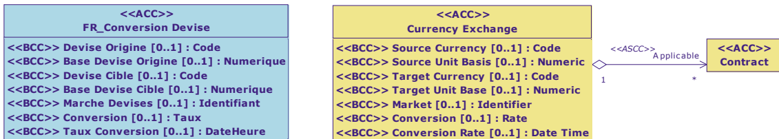
Diagramme de classe : Vue Conversion Devises
