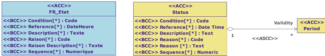
Diagramme de classe : Vue Etat
