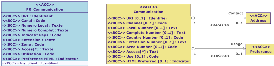
Diagramme de classe : Vue Communication
