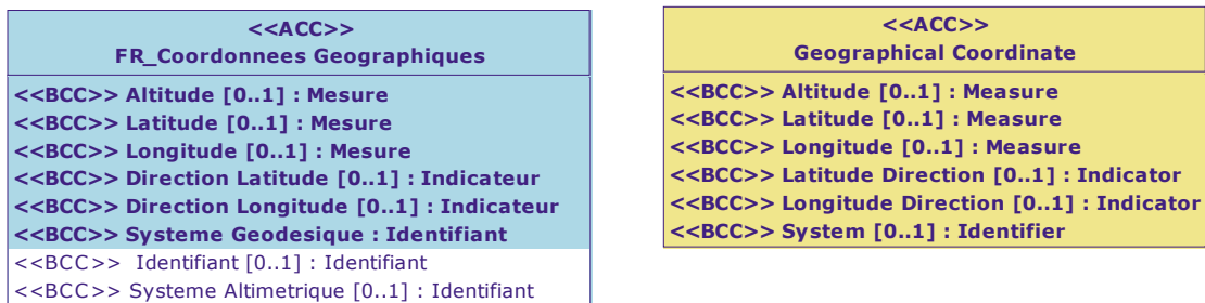
Diagramme de classe : Vue Coordonnées Géographiques
