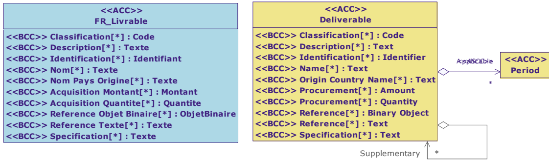
Diagramme de classe : Vue Livrable
