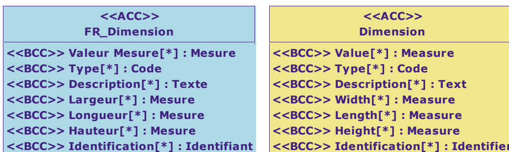
Diagramme de classe : Vue Dimension
