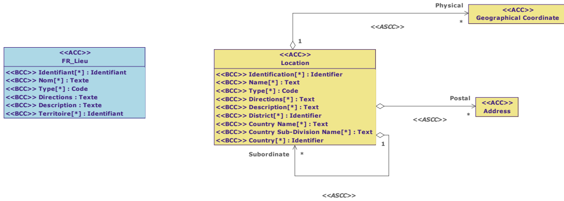
Diagramme de classe : Vue Lieu
