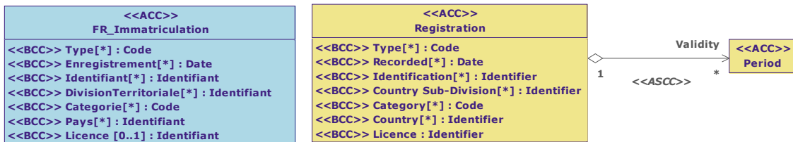
Diagramme de classe : Vue Immatriculation
