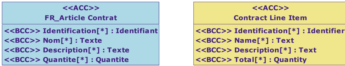
Diagramme de classe : Vue Article Contrat
