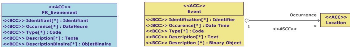
Diagramme de classe : Vue Evènement
