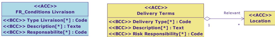
Diagramme de classe : Vue Conditions Livraison
