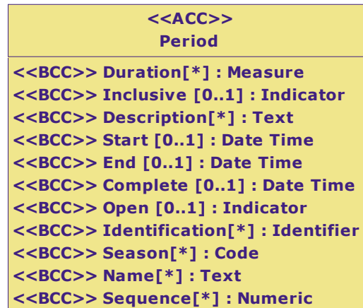
Diagramme de classe : Vue Période
