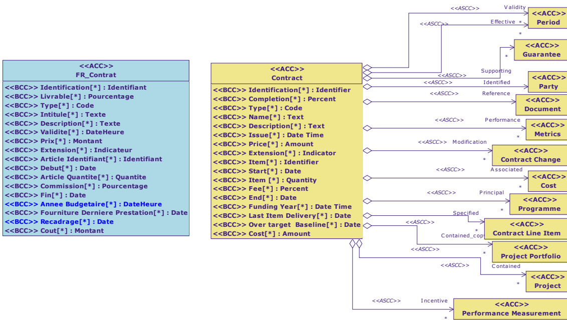
Diagramme de classe : Vue Contrat ou Marché
