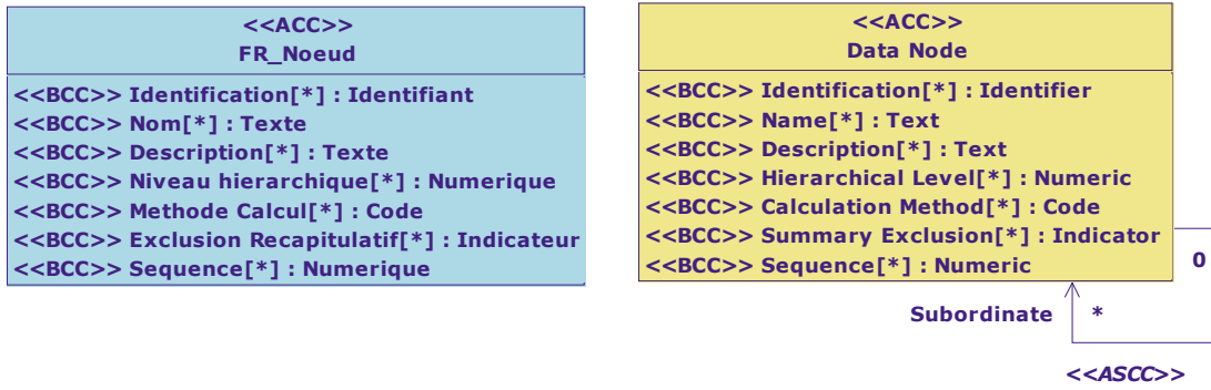
Diagramme de classe : Vue Noeud
