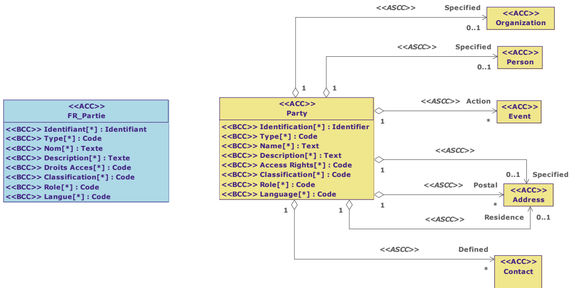
Diagramme de classe : Vue Partie
