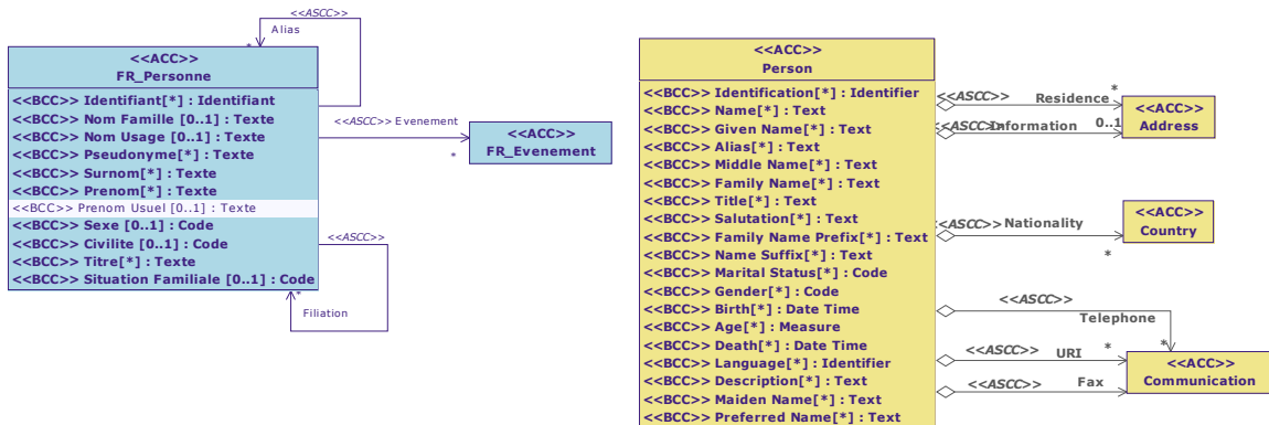
Diagramme de classe : Vue Personne
