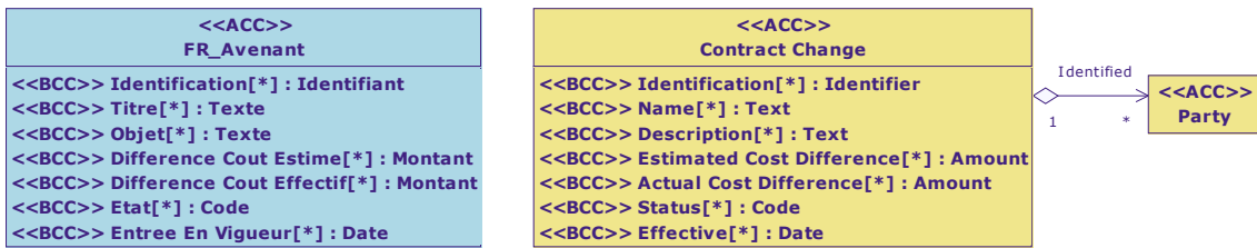
Diagramme de classe : Vue Avenant
