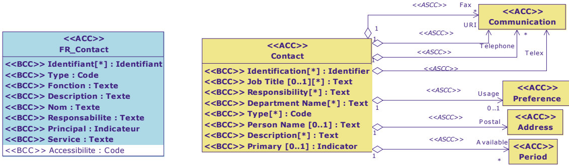
Diagramme de classe : Vue Contact
