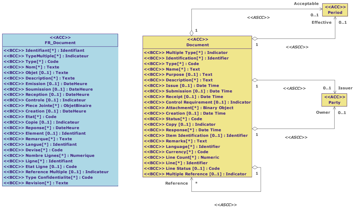
Diagramme de classe : Vue Document
