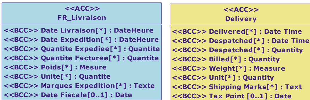
Diagramme de classe : Vue Livraison
